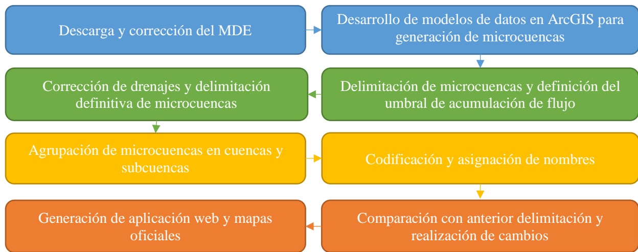
Figura 1. Esquema metodológico seguido para la delimitación de Cuencas, Subcuencas y Microcuencas
