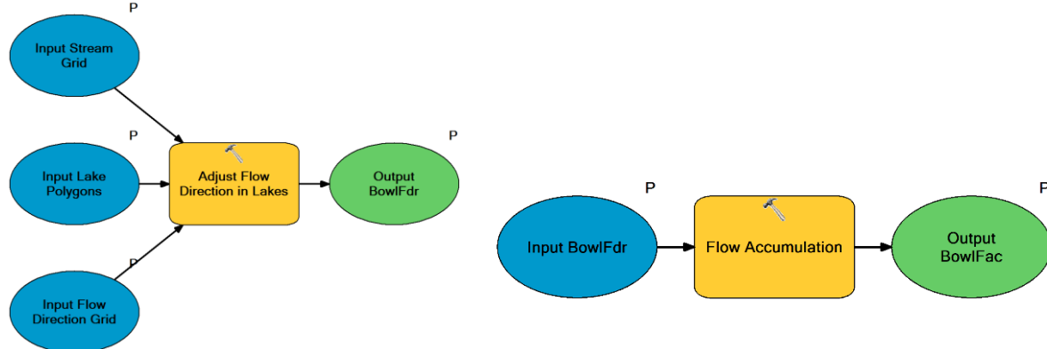
Figura 8. Modelos de datos “2_1 Ajustar Dirección de Flujo en Lagos (Opcional)” y “2_2 Generar Flujo Acumulado (Opcional)”
